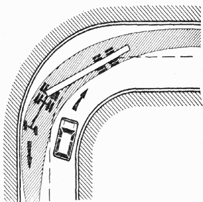
75 Поворот автопоезда с неуправляемой тележкой (занимаемая автопоездом при повороте площадь затемнена)
